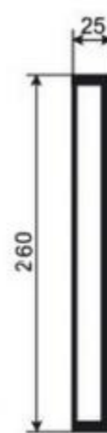
НАЛИЧНИК-МОЛДИНГ НМ-РП-17
