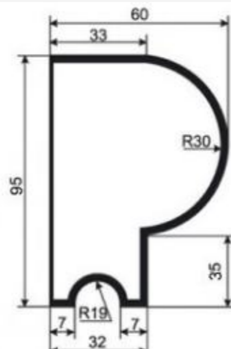
МОЛДИНГ М-РП-2
