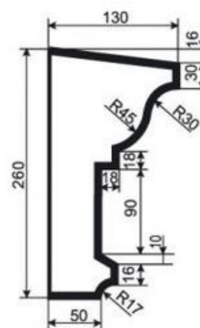
КАРНИЗ К-РП-38
