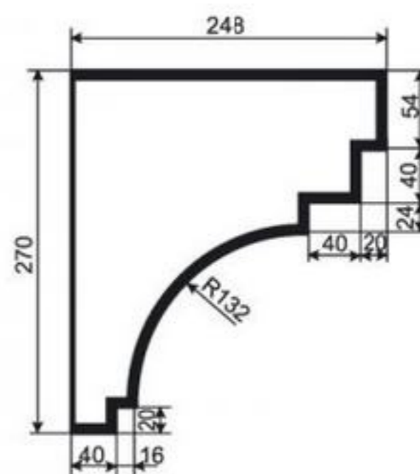
КАРНИЗ К-РП-42
