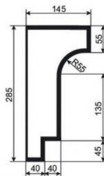
КАРНИЗ К-РП-46
