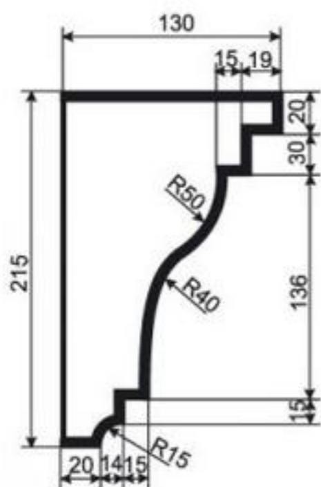
КАРНИЗ К-РП-29
