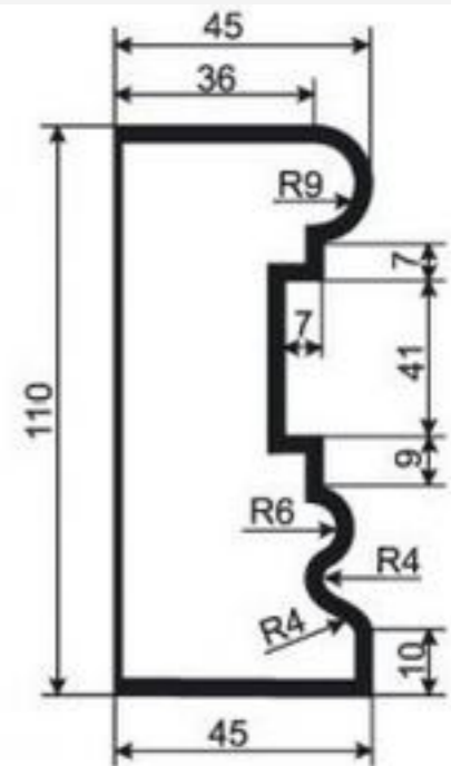
МОЛДИНГ М-РП-1
