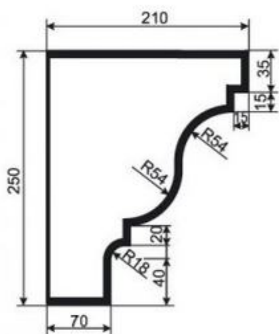
КАРНИЗ К-РП-39
