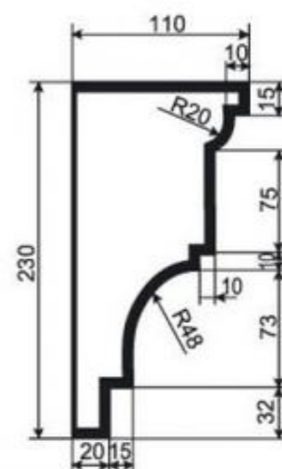
КАРНИЗ К-РП-32
