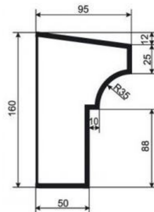
КАРНИЗ К-РП-10
