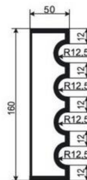
НАЛИЧНИК-МОЛДИНГ НМ-РП-11
