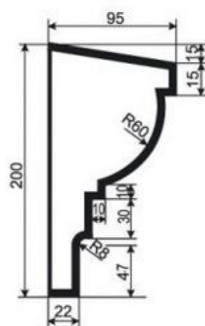
КАРНИЗ К-РП-20
