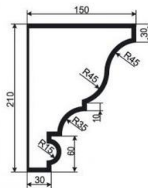
КАРНИЗ К-РП-24
