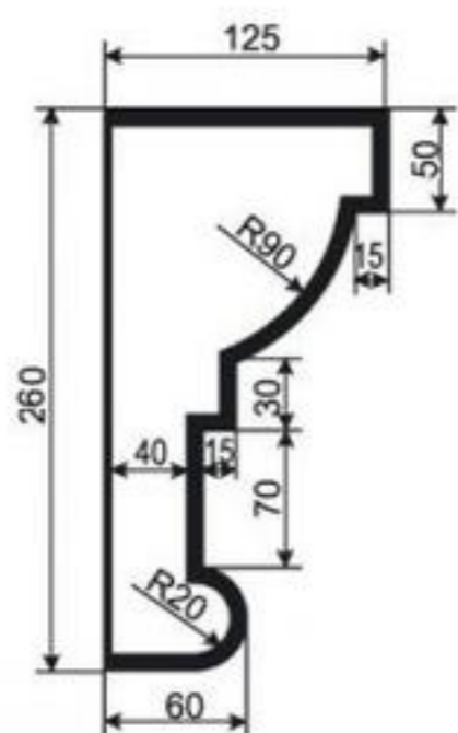
КАРНИЗ К-РП-37
