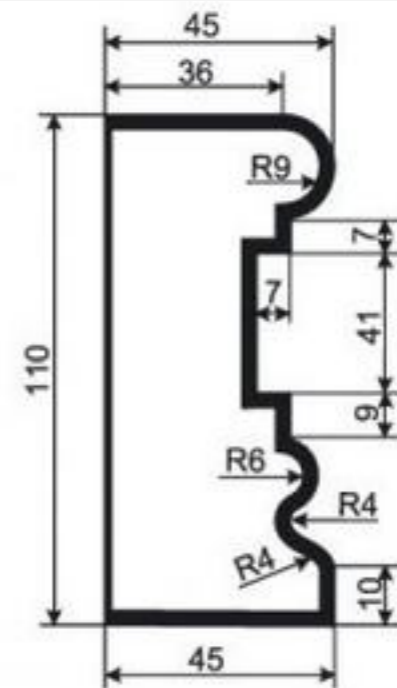
МОЛДИНГ М-РП-4
