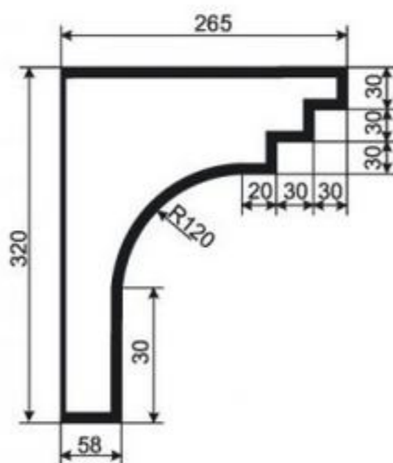
КАРНИЗ К-РП-55
