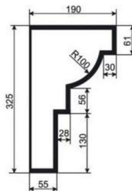
КАРНИЗ К-РП-54
