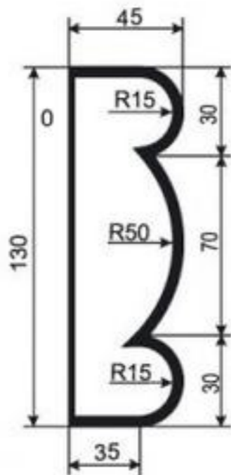
НАЛИЧНИК-МОЛДИНГ НМ-РП-4
