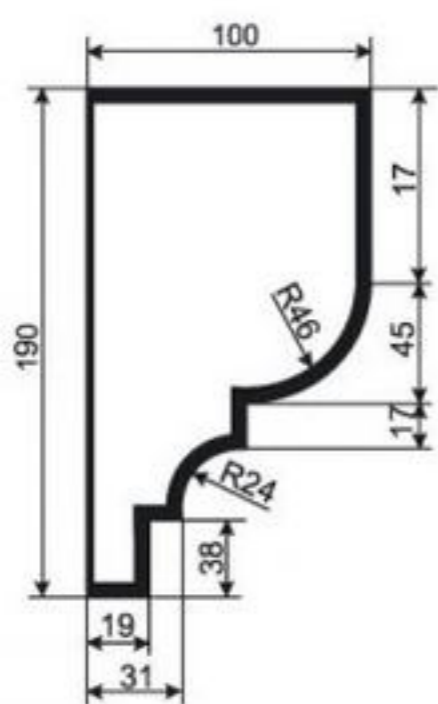
КАРНИЗ К-РП-15
