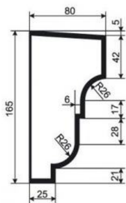
КАРНИЗ К-РП-65
