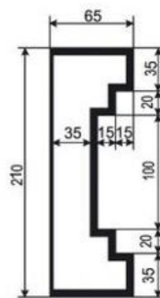
НАЛИЧНИК-МОЛДИНГ НМ-РП-15
