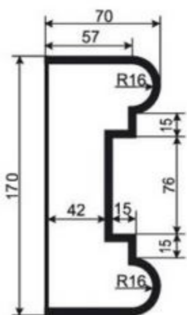
НАЛИЧНИК-МОЛДИНГ НМ-РП-12
