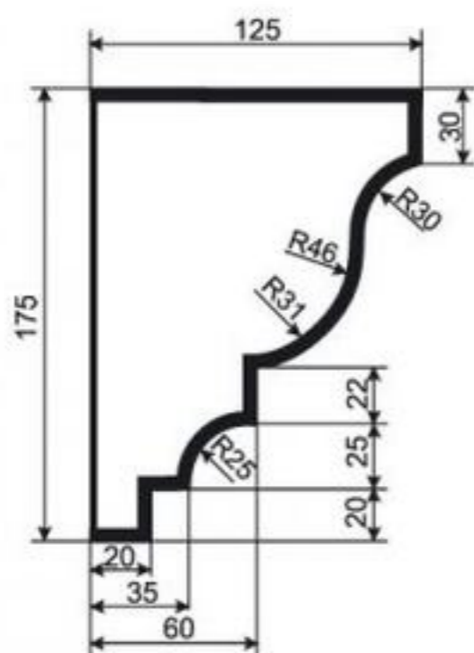
КАРНИЗ К-РП-13
