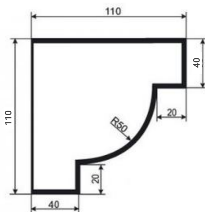
КАРНИЗ К-РП-1
