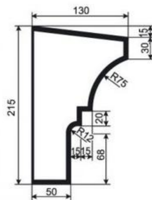
КАРНИЗ К-РП-28
