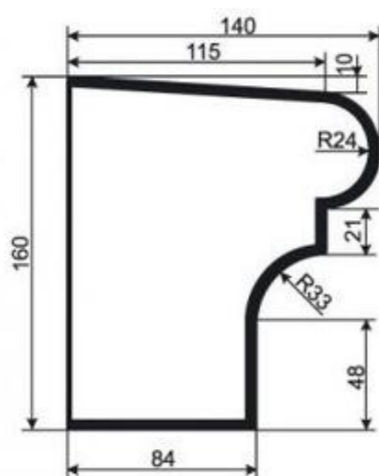
КАРНИЗ К-РП-63
