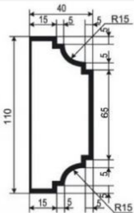
МОЛДИНГ М-РП-3
