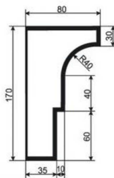
КАРНИЗ К-РП-64
