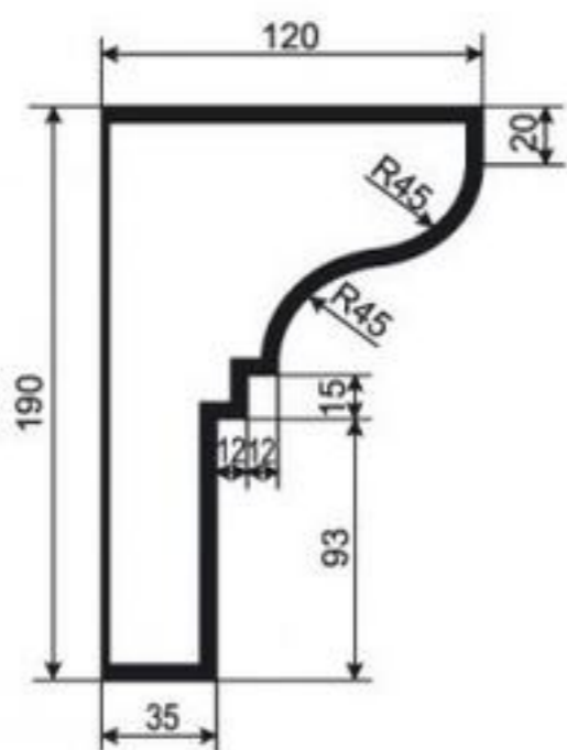
КАРНИЗ К-РП-17
