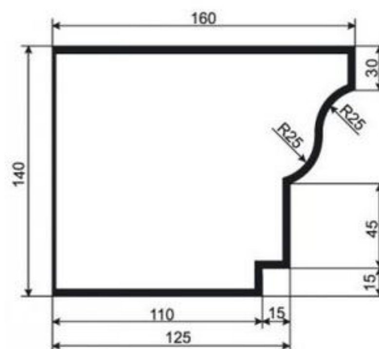
КАРНИЗ К-РП-60
