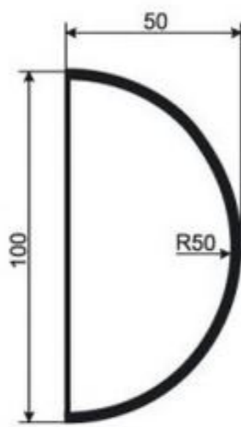
МОЛДИНГ М-РП-5
