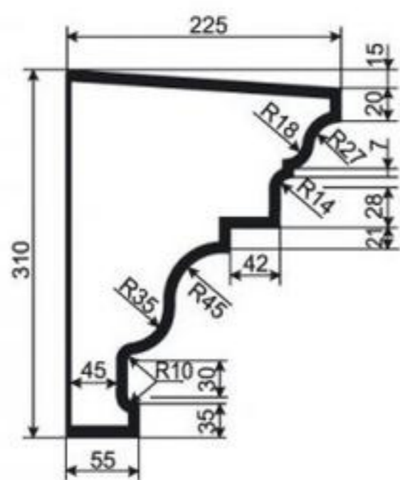
КАРНИЗ К-РП-53
