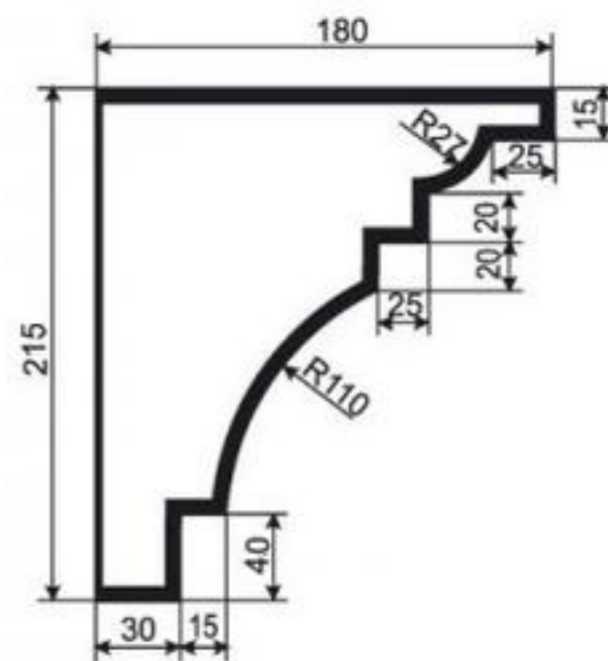
КАРНИЗ К-РП-26
