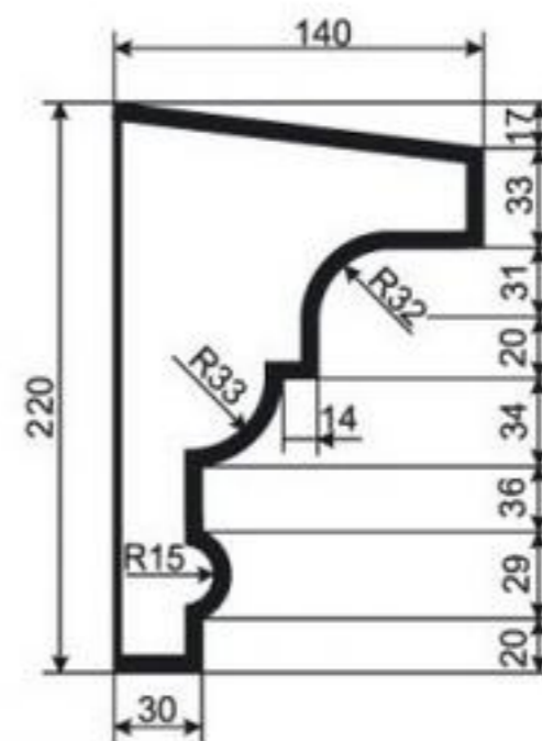
КАРНИЗ К-РП-70
