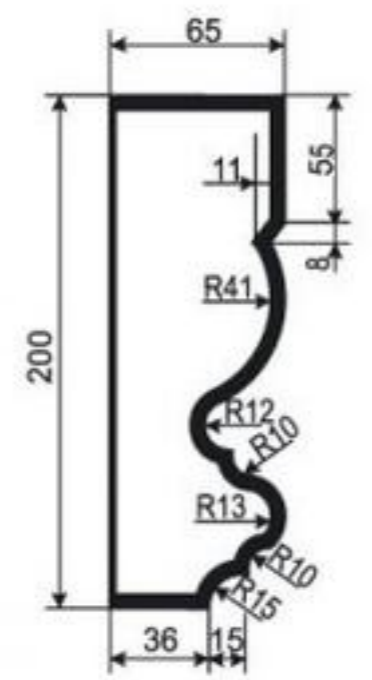
МОЛДИНГ М-РП-21
