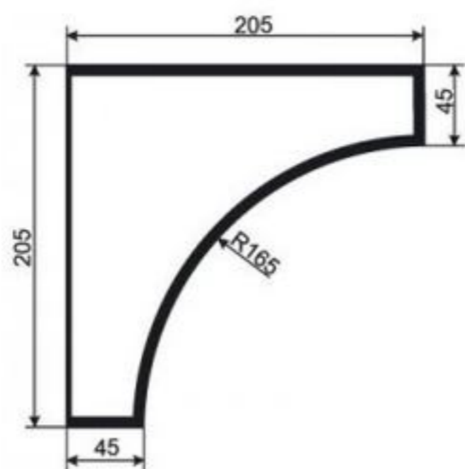
КАРНИЗ К-РП-27
