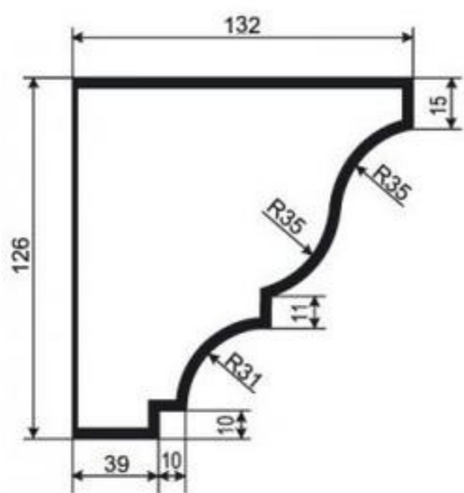
КАРНИЗ К-РП-3
