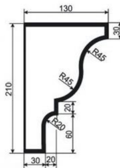
КАРНИЗ К-РП-22
