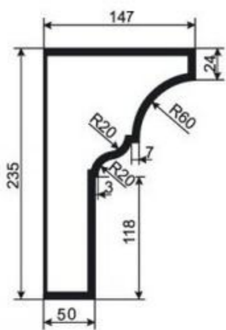
КАРНИЗ К-РП-35
