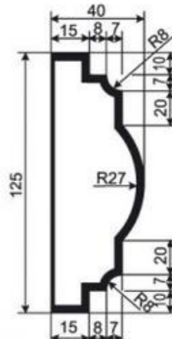
МОЛДИНГ М-РП-8
