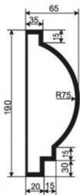
МОЛДИНГ М-РП-11
