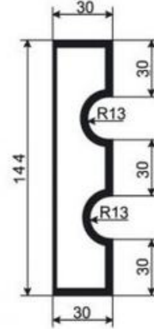
НАЛИЧНИК-МОЛДИНГ НМ-РП-5
