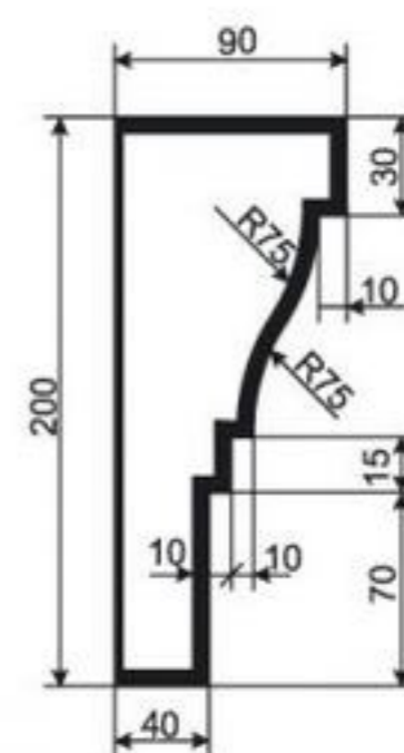
КАРНИЗ К-РП-68
