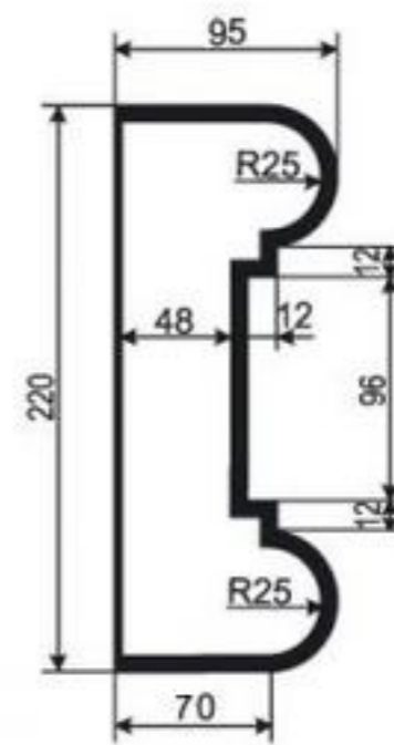
МОЛДИНГ М-РП-24
