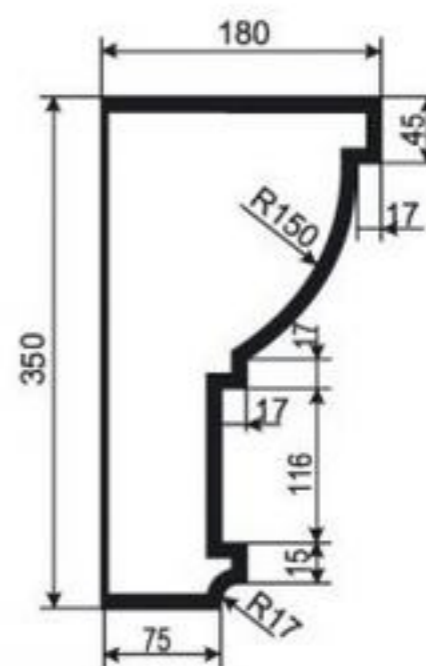
КАРНИЗ К-РП-56
