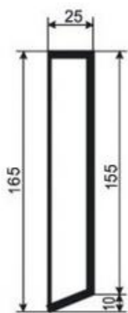
НАЛИЧНИК-МОЛДИНГ НМ-РП-10
