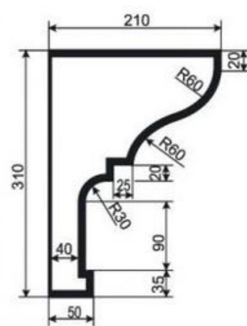
КАРНИЗ К-РП-52
