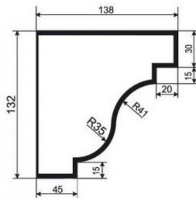
КАРНИЗ К-РП-4
