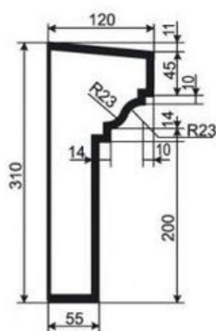
КАРНИЗ К-РП-49
