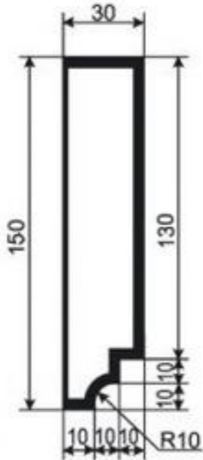
НАЛИЧНИК-МОЛДИНГ НМ-РП-6
