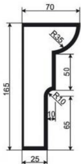
МОЛДИНГ М-РП-15
