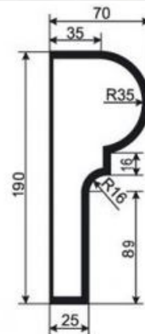
МОЛДИНГ М-РП-18
