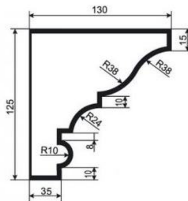
КАРНИЗ К-РП-2
