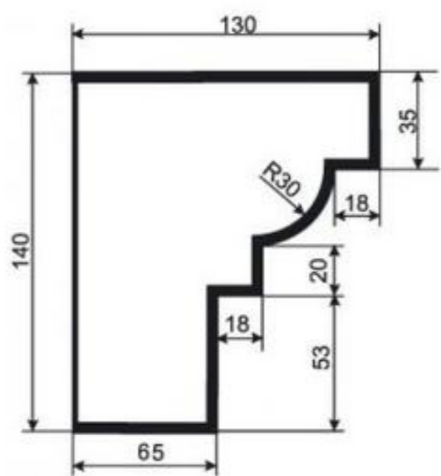
КАРНИЗ К-РП-5
