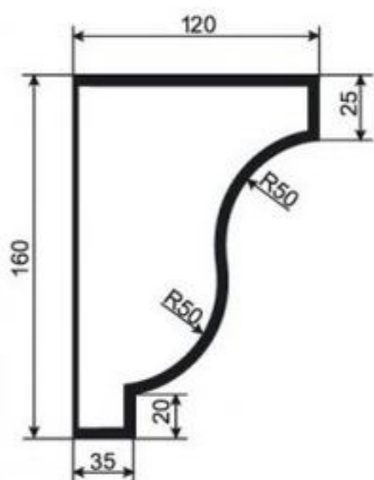
КАРНИЗ К-РП-11
