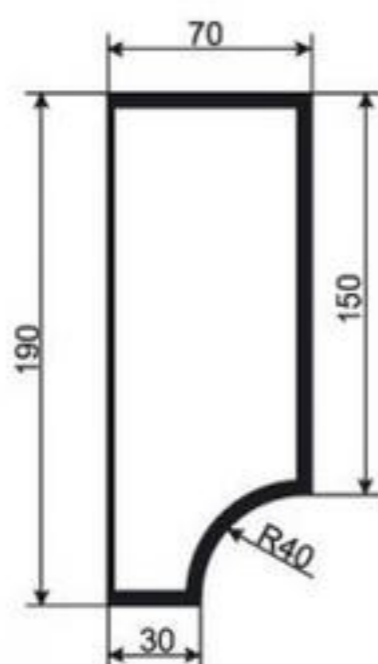
НАЛИЧНИК-МОЛДИНГ НМ-РП-14
