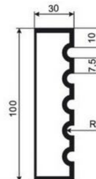
НАЛИЧНИК-МОЛДИНГ НМ-РП-1
