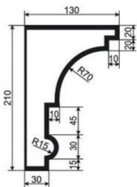
КАРНИЗ К-РП-23
