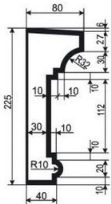
МОЛДИНГ М-РП-23
