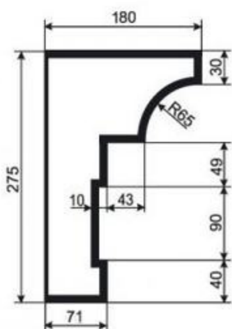
КАРНИЗ К-РП-43
