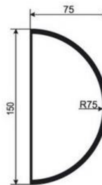
НАЛИЧНИК-МОЛДИНГ НМ-РП-9
