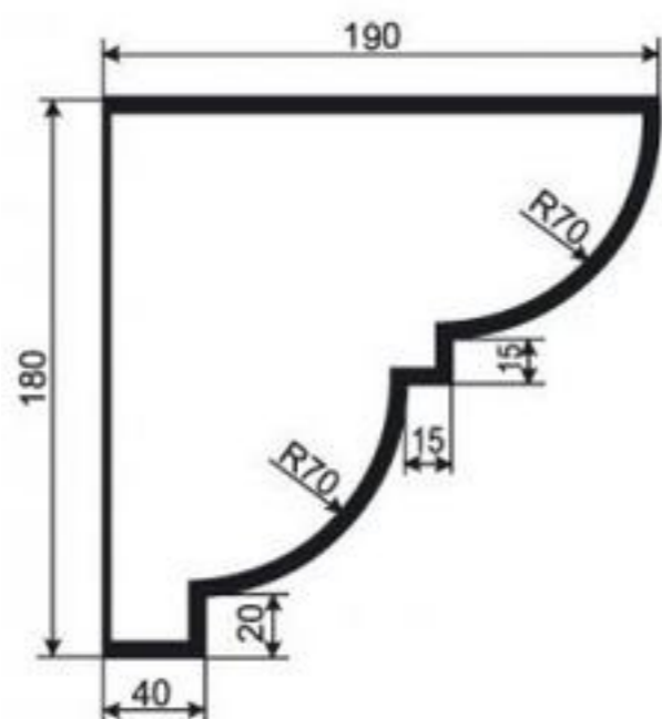
КАРНИЗ К-РП-19
