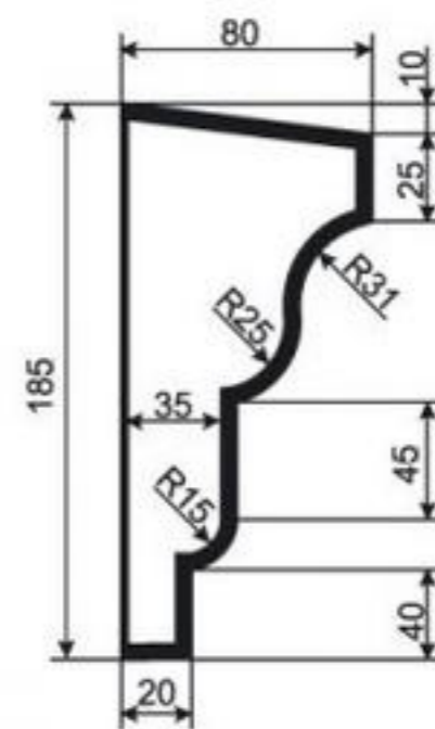
КАРНИЗ К-РП-66
