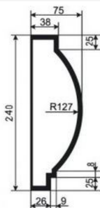
НАЛИЧНИК-МОЛДИНГ НМ-РП-16
