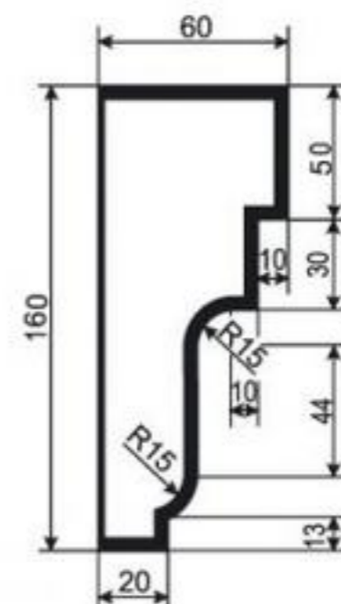
МОЛДИНГ М-РП-14
