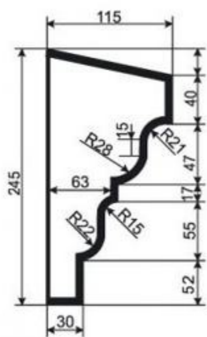
КАРНИЗ К-РП-71
