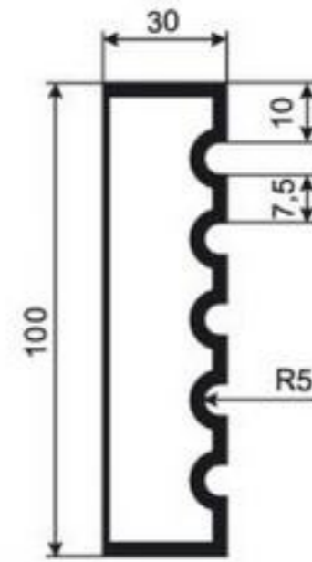
МОЛДИНГ М-РП-6
