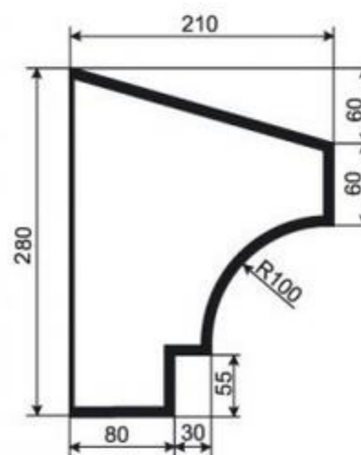
КАРНИЗ К-РП-44
