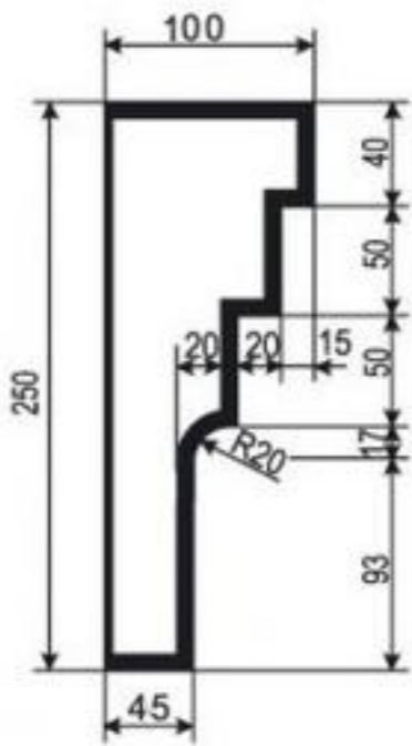
МОЛДИНГ М-РП-25
