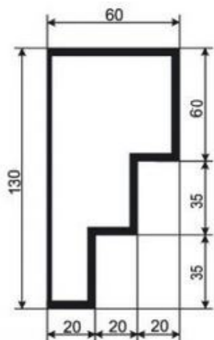
МОЛДИНГ М-РП-9
