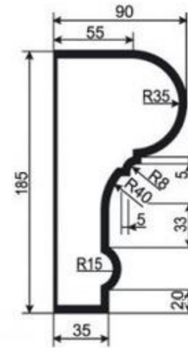
МОЛДИНГ М-РП-20
