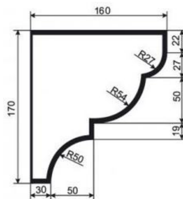
КАРНИЗ К-РП-14
