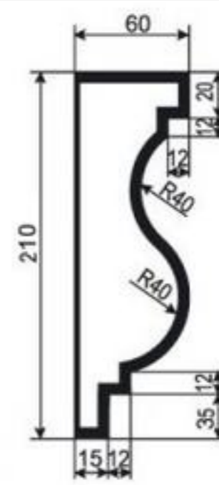
МОЛДИНГ М-РП-22
