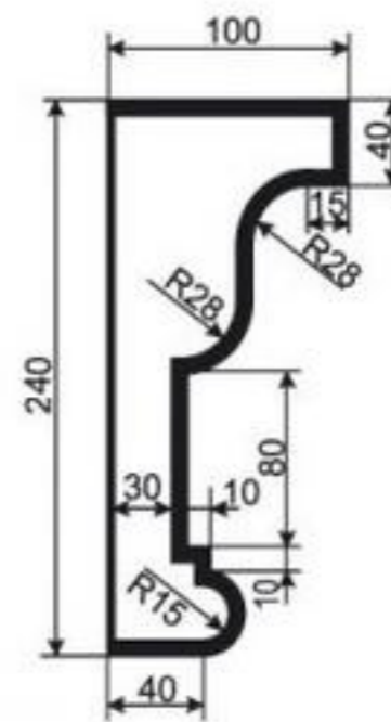
КАРНИЗ К-РП-34
