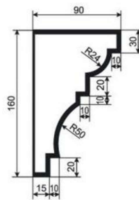
КАРНИЗ К-РП-8
