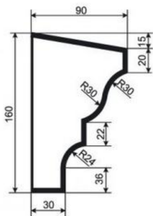
КАРНИЗ К-РП-9
